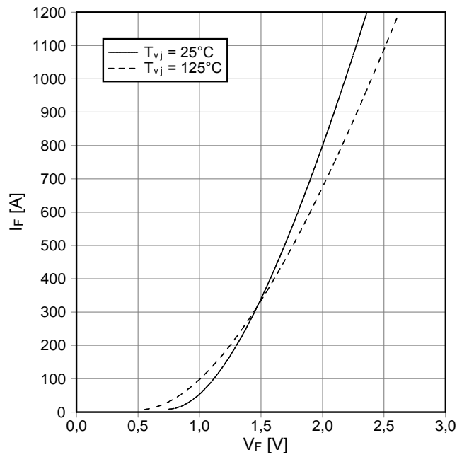
Durchlaßkennlinie der Diode-Wechselr. (typisch) forward characteristic of diode-inverter (typical) I_F = f(V_F)
